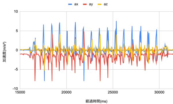
図 12: 加速度センサデータ（履き口外側装着時）
