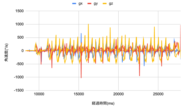
図 16: ジャイロセンサデータ（履き口内側装着時）
