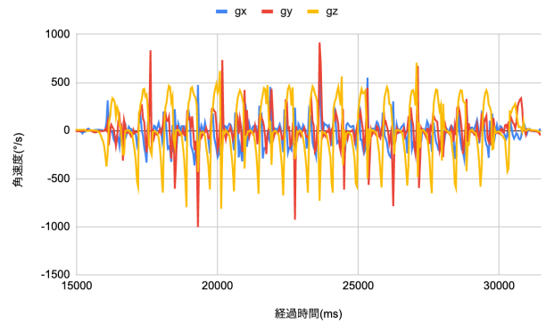
図 15: ジャイロセンサデータ（履き口外側装着時）
