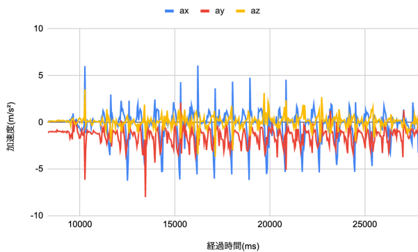
図 13: 加速度センサデータ（履き口内側装着時）
