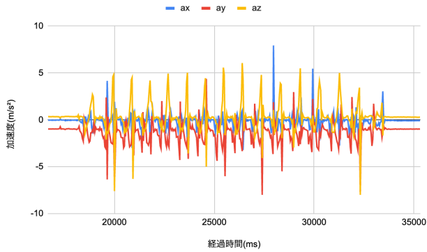
図 11: 加速度センサデータ（踵装着時）
