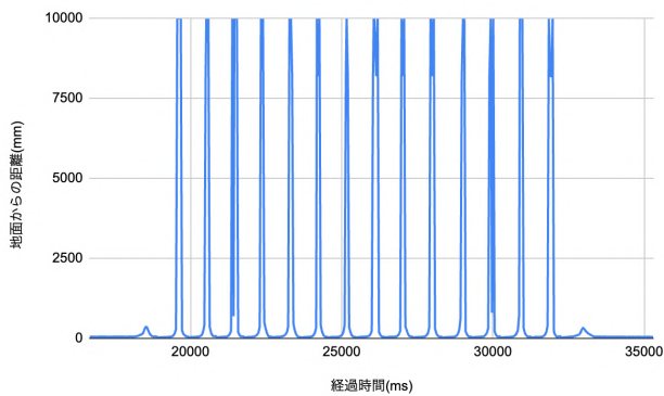
図 17: 測距センサデータ（踵装着時）
