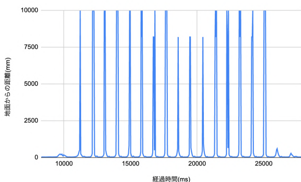
図 19: 測距センサデータ（履き口内側装着時）
