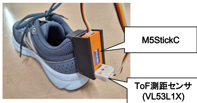
図 4: 靴装着型デバイスの外観の図
