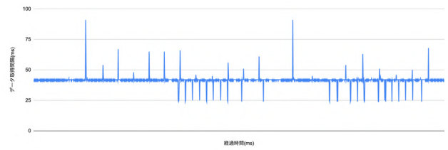
図 8: データ取得間隔（踵装着時）
