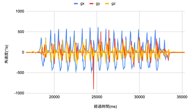
図 14: ジャイロセンサデータ（踵装着時）
